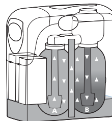
La colonne A est en régénération La colonne B adoucit
